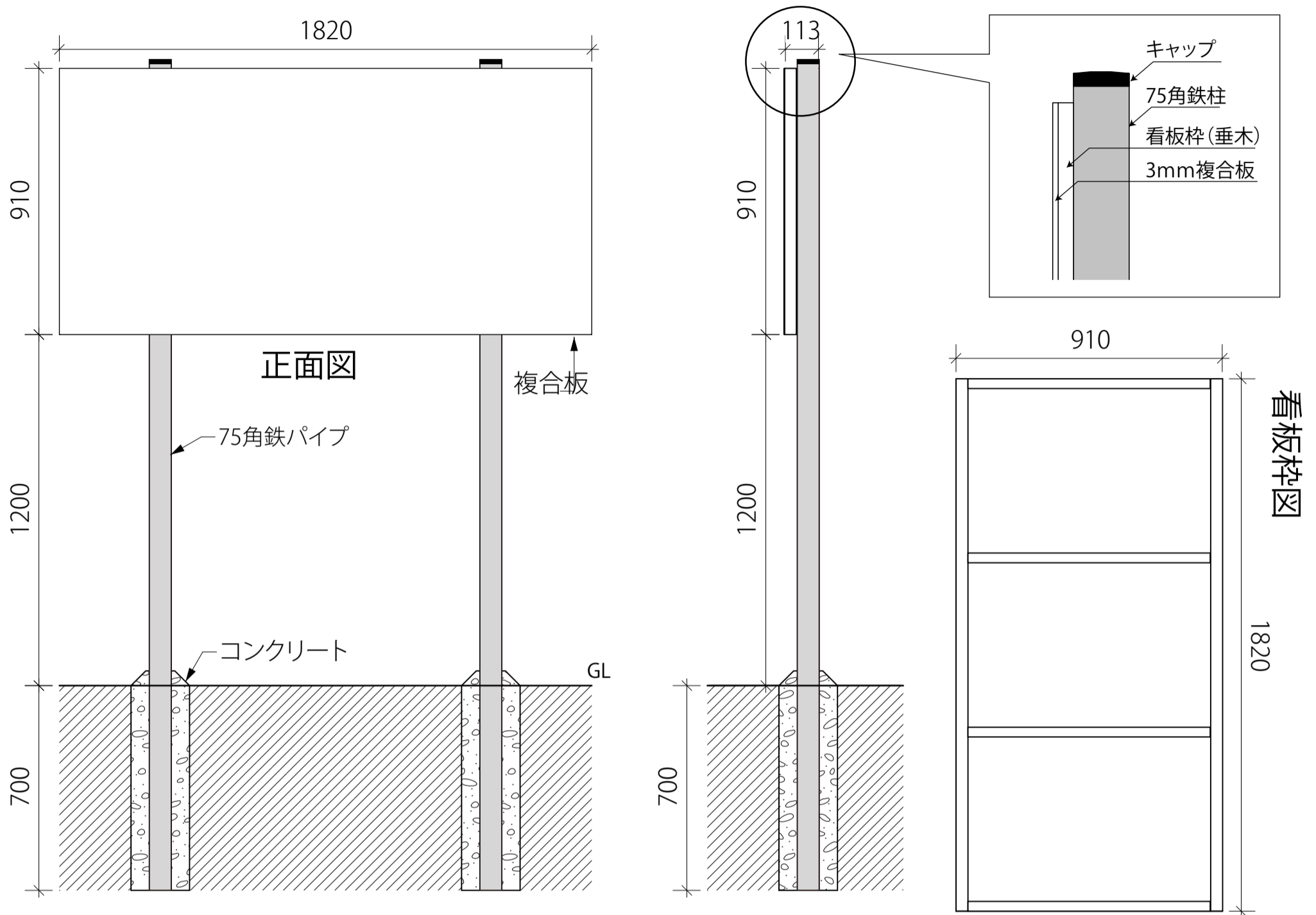
看板見本 1820mm
